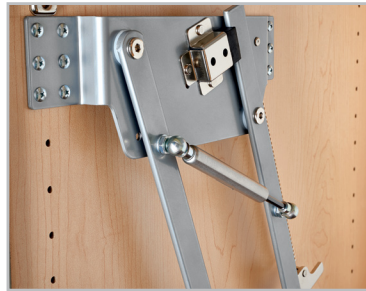
Soft-Close piston
